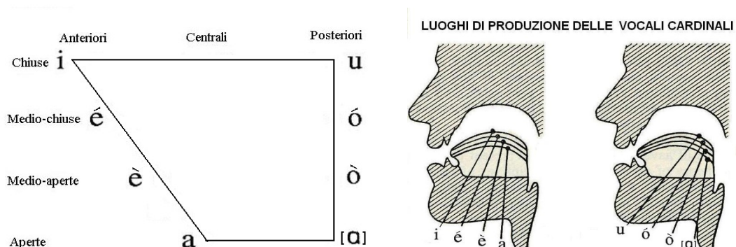
Fig. 1 . Diagramma dei suoni vocalici della lingua italiana.
