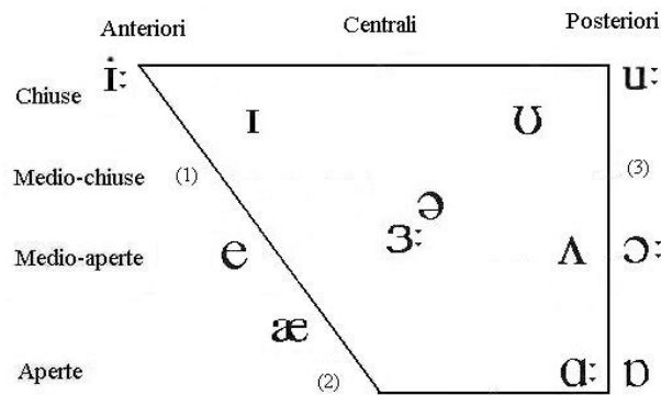
Fig. 2 . Diagramma dei suoni vocalici inglesi "critici".
